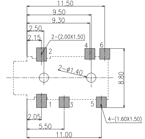
P.C.B LAYOUT
